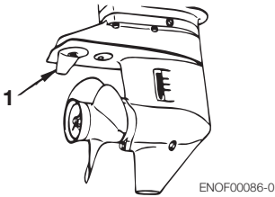
1. Anode (Trimmflosse)
