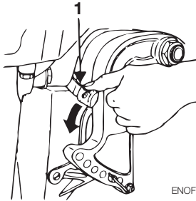
1. Rückfahrsperrhebel
