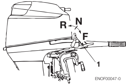
1. Schalthebel
